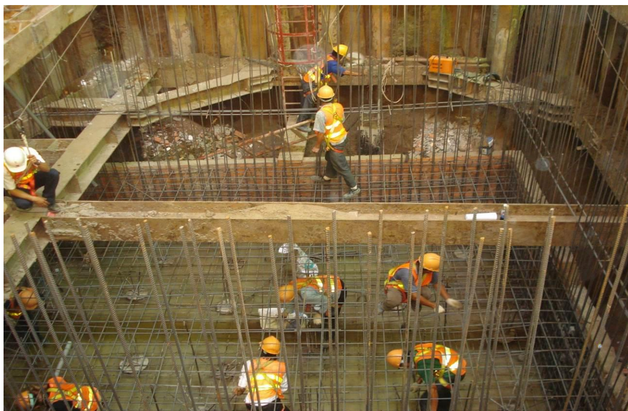
THI CÔNG MÓNG MÁY – CỪ LARSEN & HỆ GIÀNG THÉP
