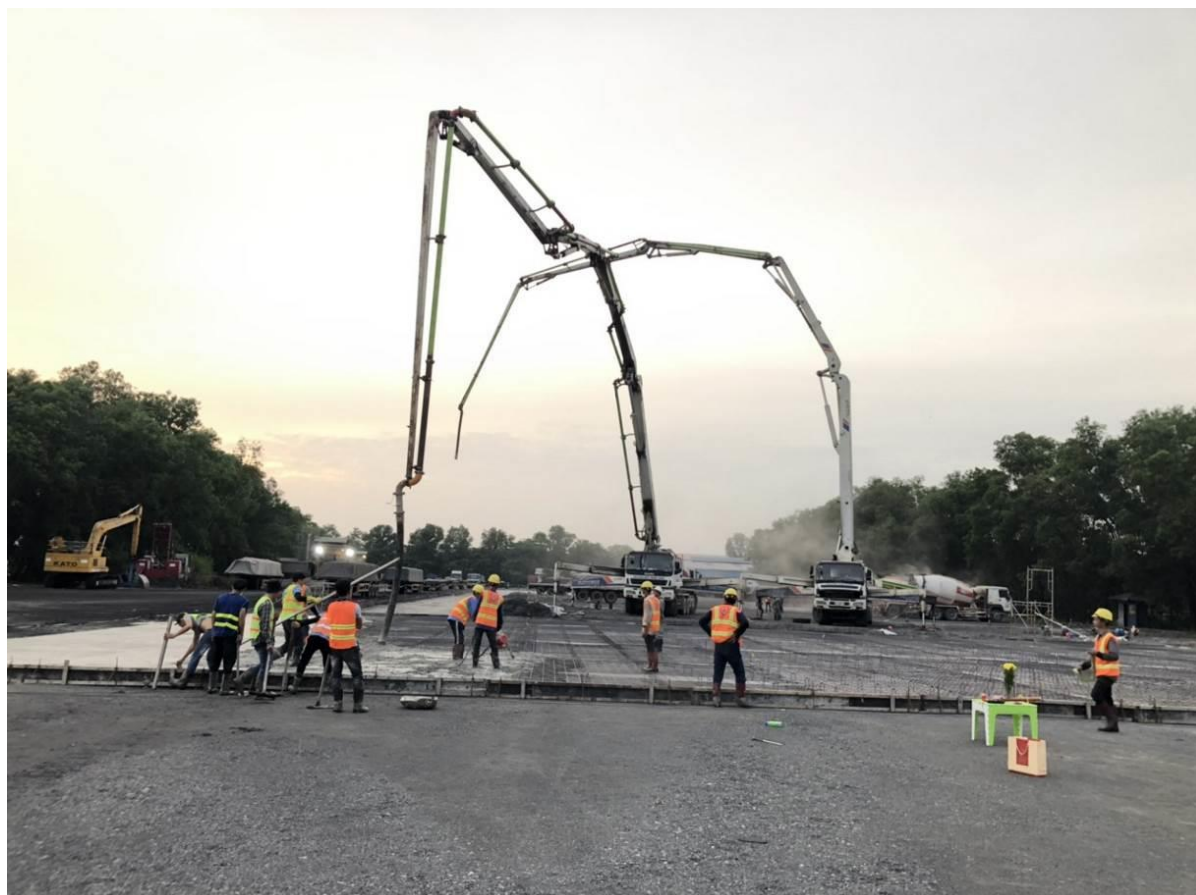
XÂY DỰNG HẠ TẦNG CẢNG BẾN KÉO – FICO YTL - TÂY NINH INFRASTRUCTURE OF BEN KEO JETTY – FICO YTL - TAY NINH
