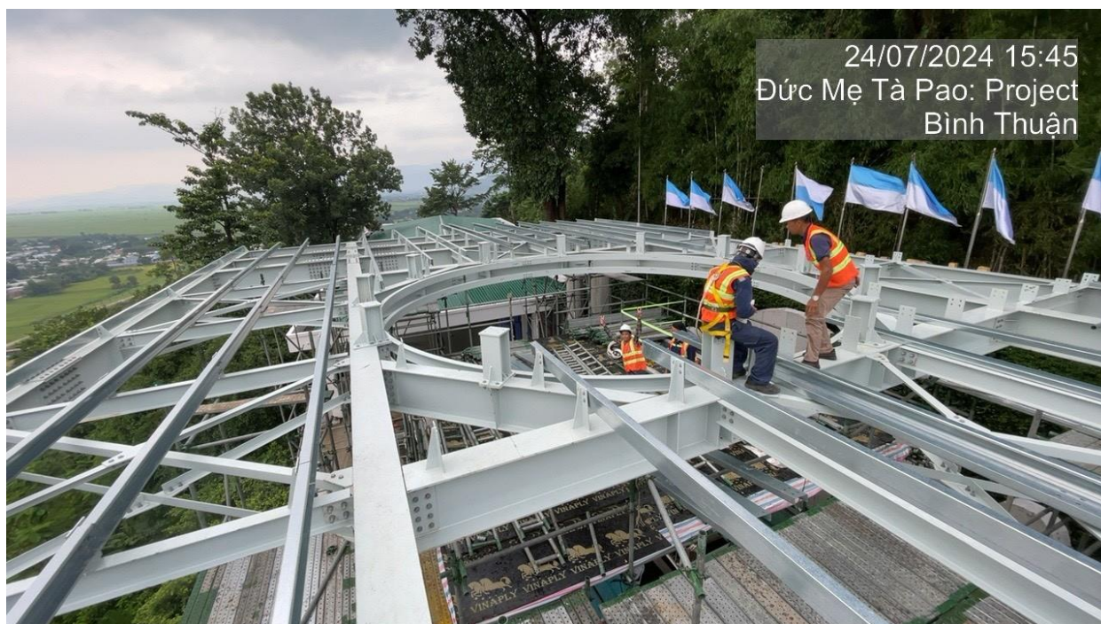
LẮP DỰNG KẾT CẤU THÉP MÁI CHE LINH ĐÀI ĐỨC MẸ TÀPAO:
