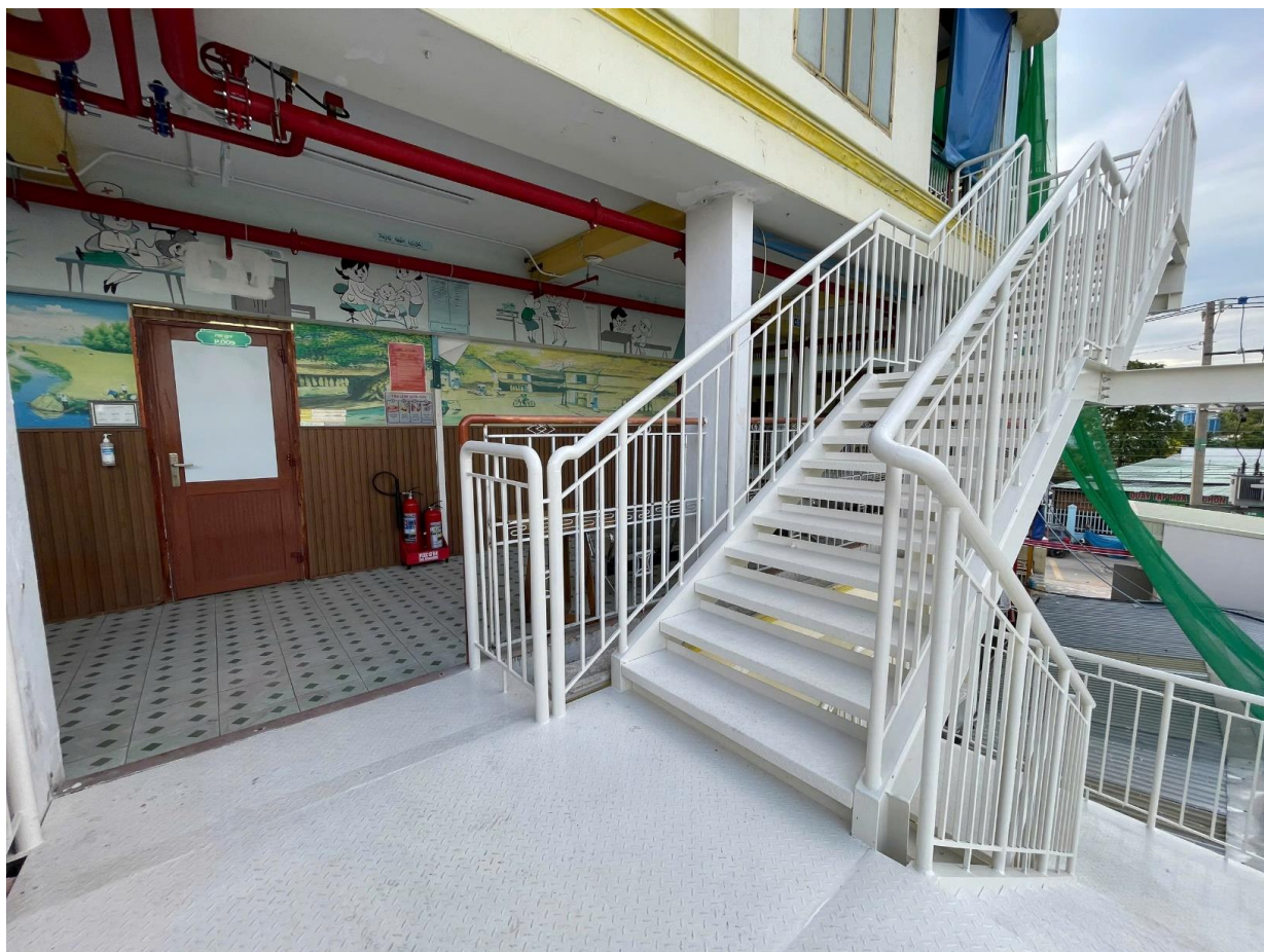
DỰ ÁN: BỆNH VIỆN HOÀN MỸ BÌNH DƯƠNG HẠNG MỤC: CẦU THANG THOÁT HIỂM, BỂ NƯỚC PCCC, NHÀ BƠM
