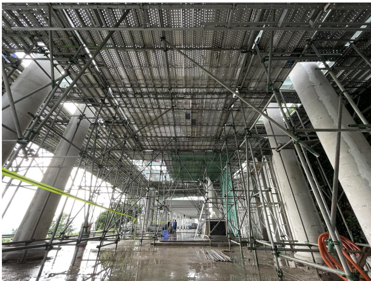
GIÀN GIÁO AN TOÀN BS1139 ĐỂ THI CÔNG KẾT CẤU THÉP
